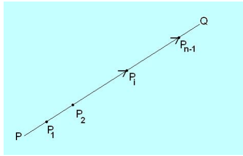
Figure 1: Coordenadas de P_i .
