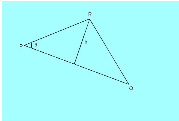
Figure 2: Triángulo en \mathcal{E}_n .
