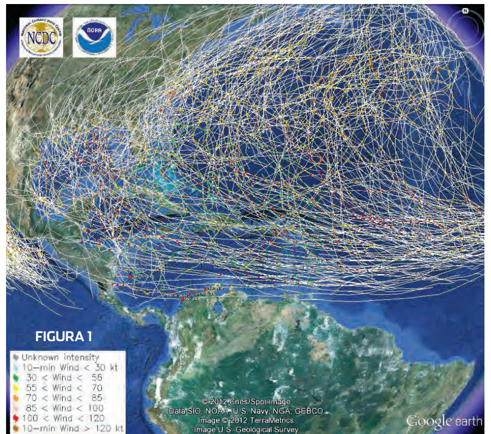
Trayectoria de los huracanes que han cruzado el Caribe colombiano (Tomado de Google Earth y HURdata de NOAA).
